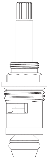
Cabeza Transferencia Novara / Lucca / Toscana
