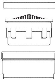
Porta boquilla macho M21,5 - Aireador - Sello de goma CODIGO: R20
