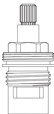
Cabeza Cerámica Novara / Lucca / Toscana Cocina / Ducha Ext.
