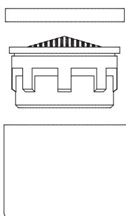
Porta boquilla hembra M21,5 - Aireador - Sello de goma CODIGO: 1690061
