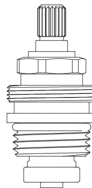
Cabeza compresión Ducha exterior
